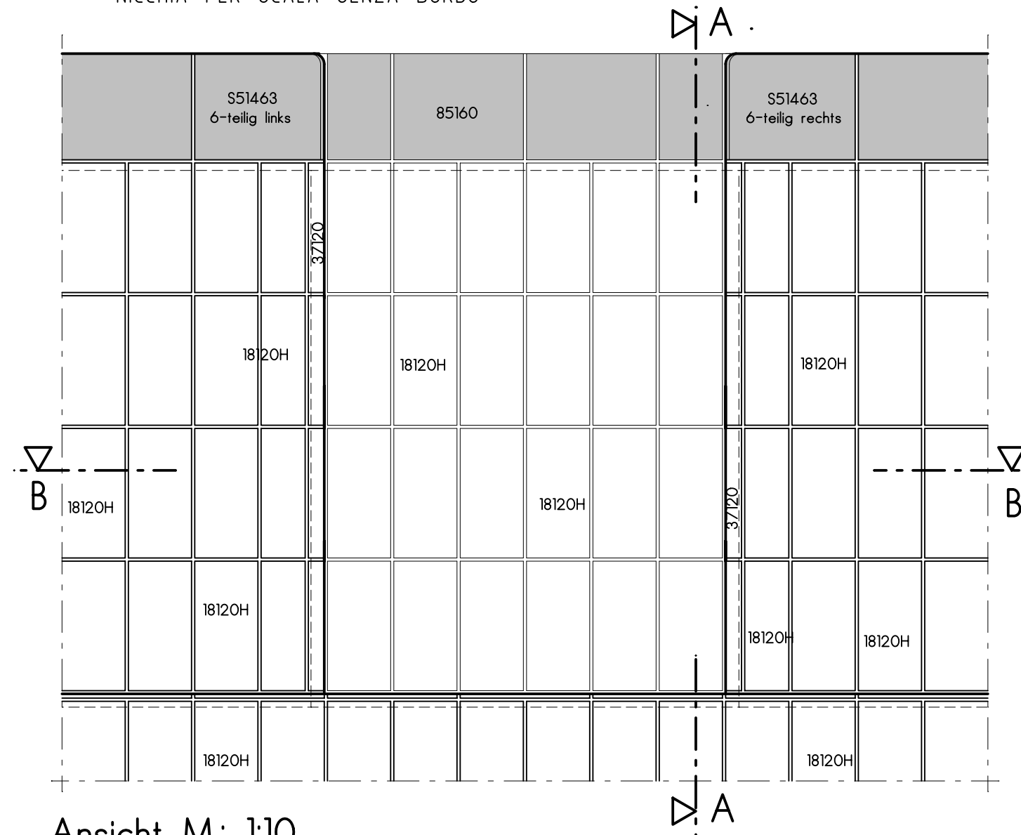
Ansicht M.: 1:10 VUE / VIEW / VISTA
