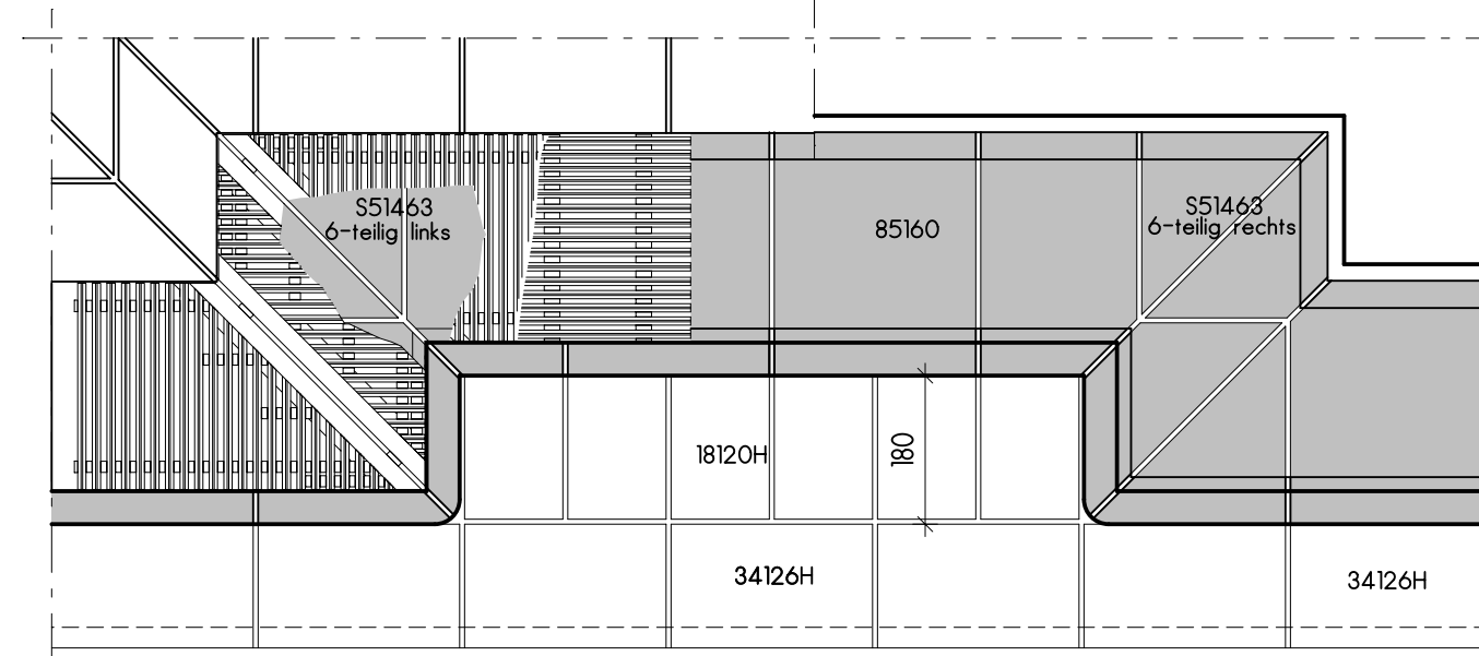
Draufsicht VUE D'EN HAUT / TOP VIEW / VISTA DALL'ALTO
