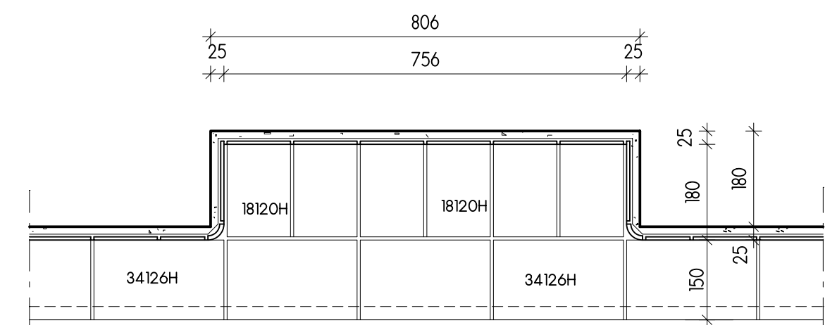
Schnitt B-B COUPE B-B / SECTION B-B / SEZIONE B-B
