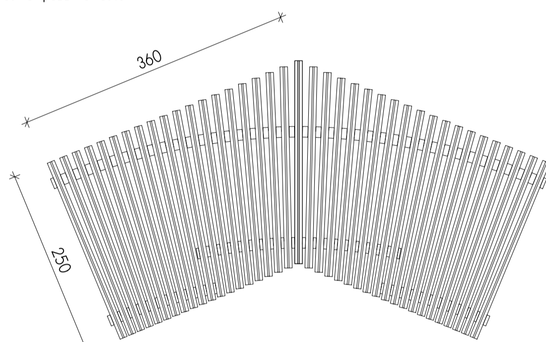
Fächerecke 135°-179°
