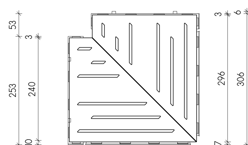
Außenecke
