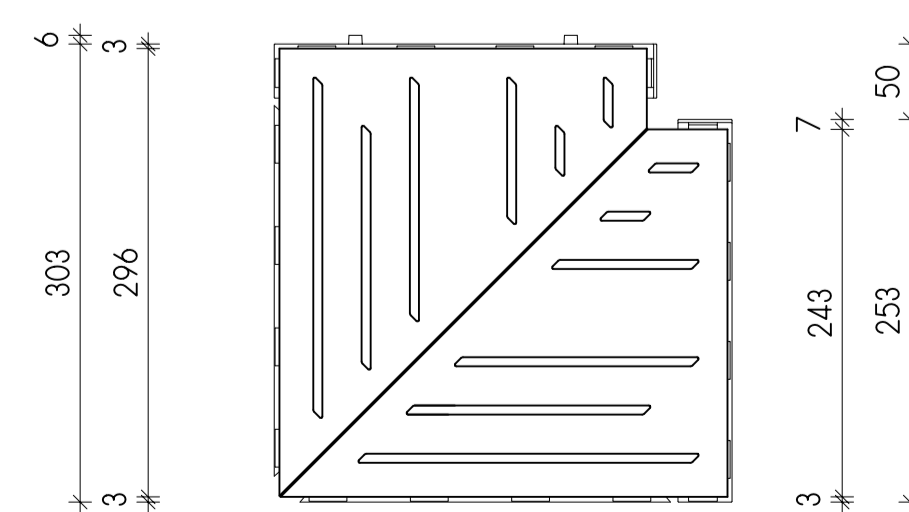
Innenecke
