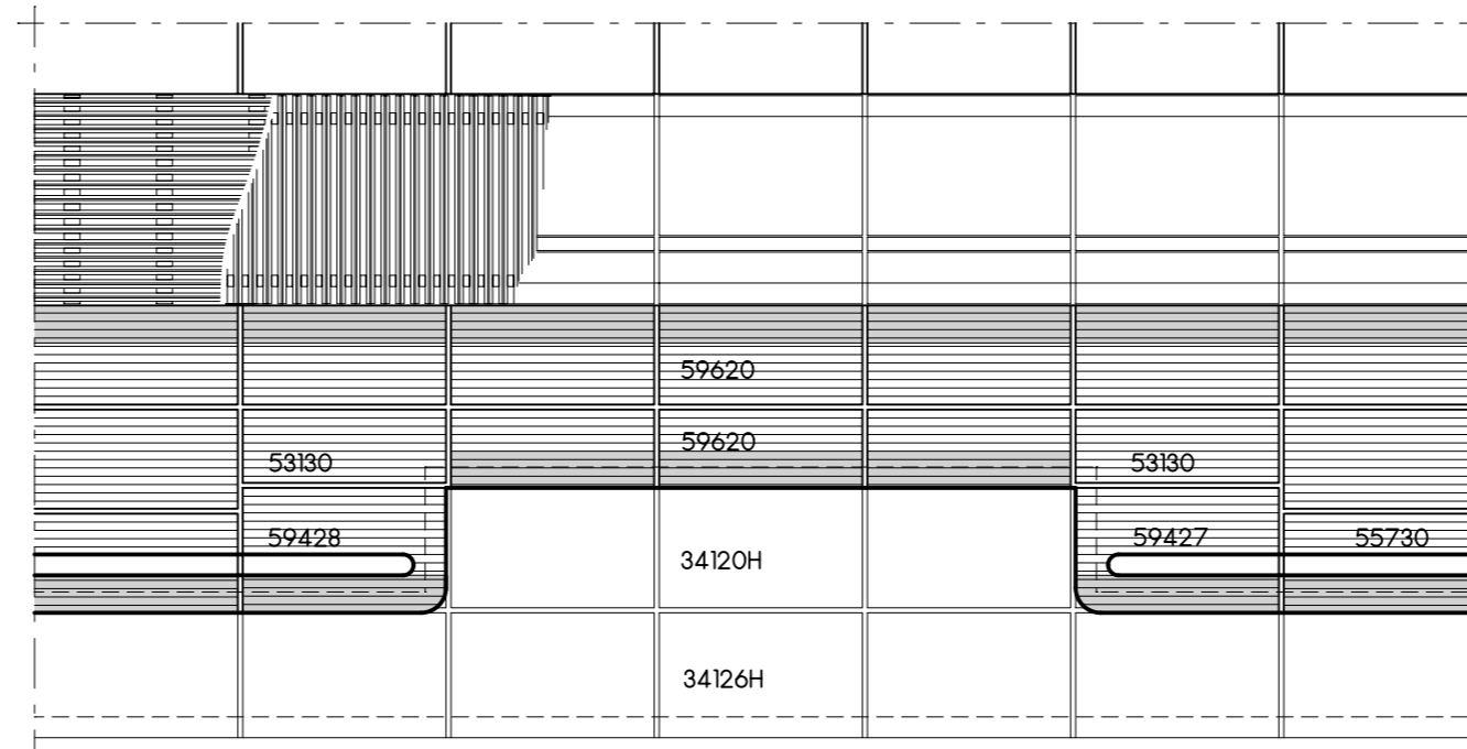
ANSICHT VUE / VIEW / VISTA
