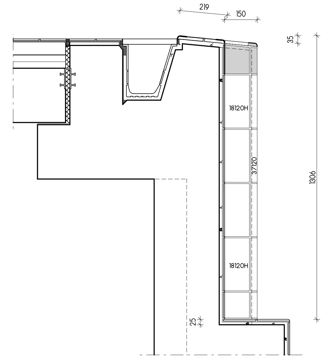
SCHNITT A-A COUPE A-A / SECTION A-A / SEZIONE A-A
